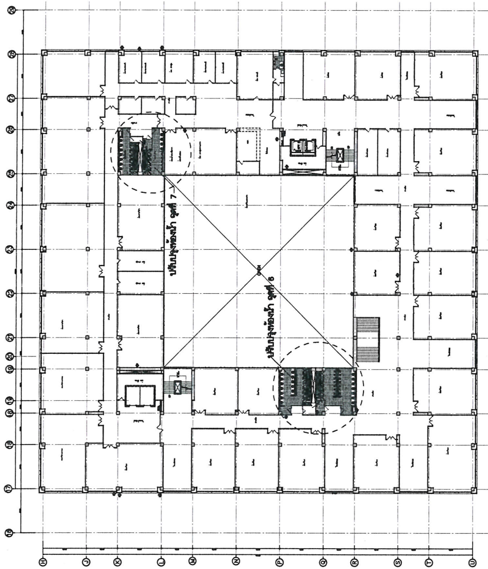
แปลนแสดงตำแหน่งห้องน้ำที่ปรับปรุง ชั้นที่ 3
